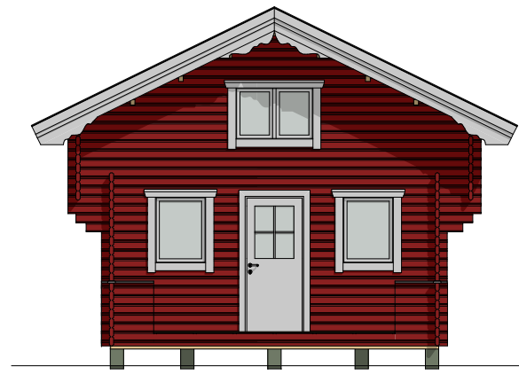
A2 Fasad 1:100
