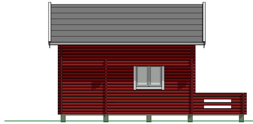
A1 Fasad 1:100
