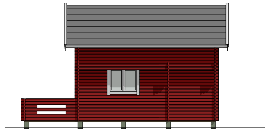
A3 Fasad 1:100
