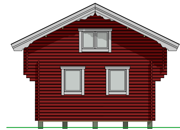
A4 Fasad 1:100
