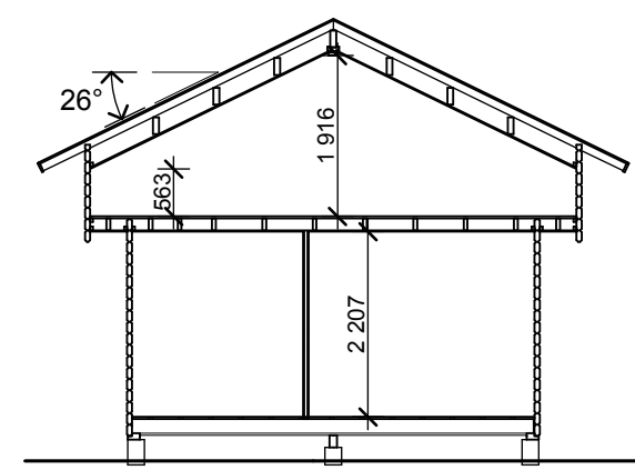
S3 1:100
